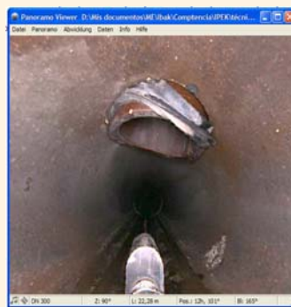
Acometida sobresaliente
